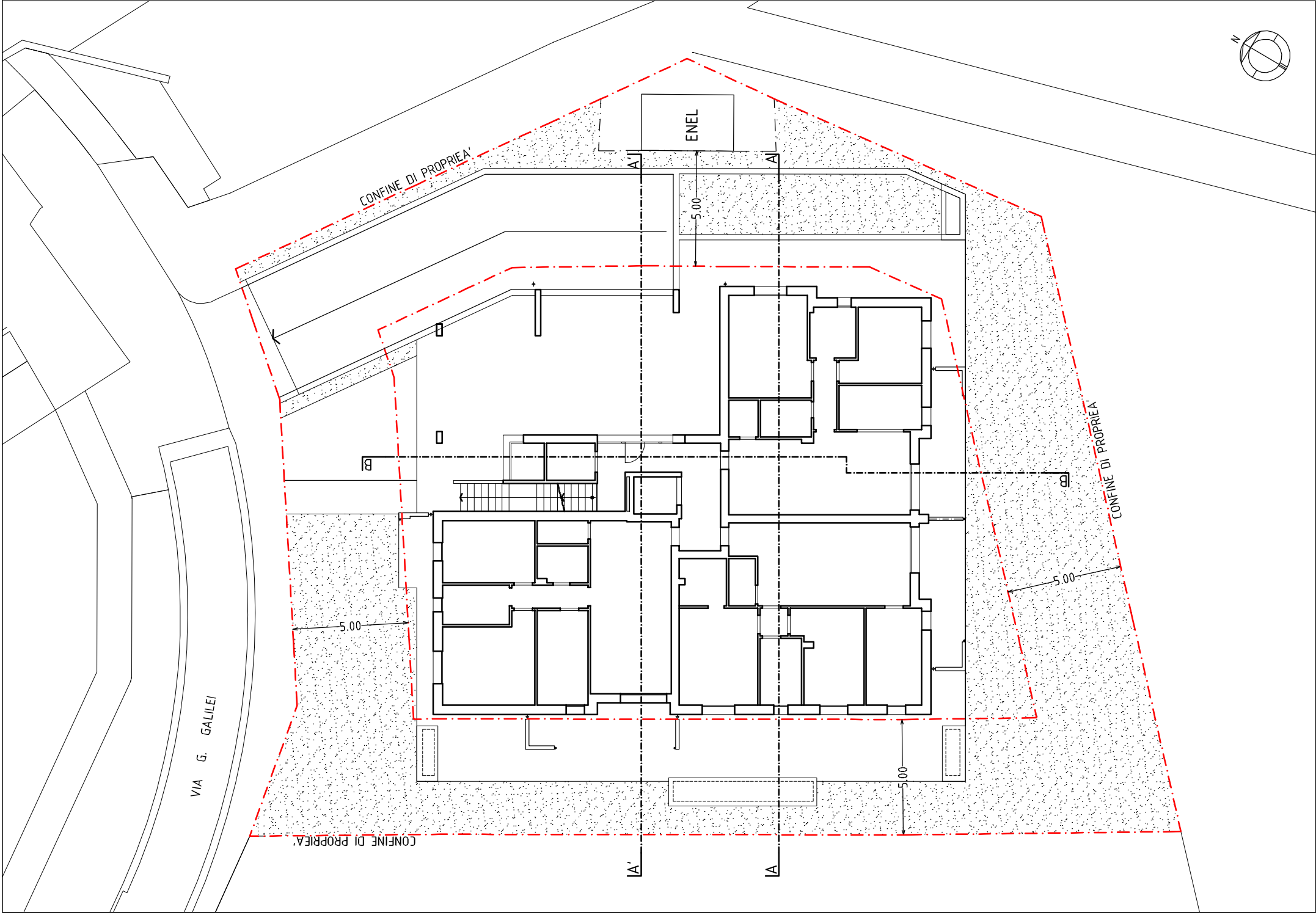
PLANIMETRIA G. PIANTA P. TERRENO
