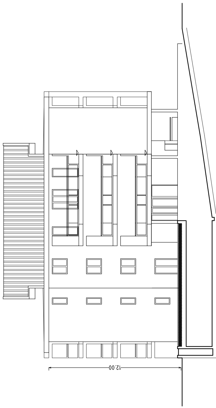
PROSPETTO EST
