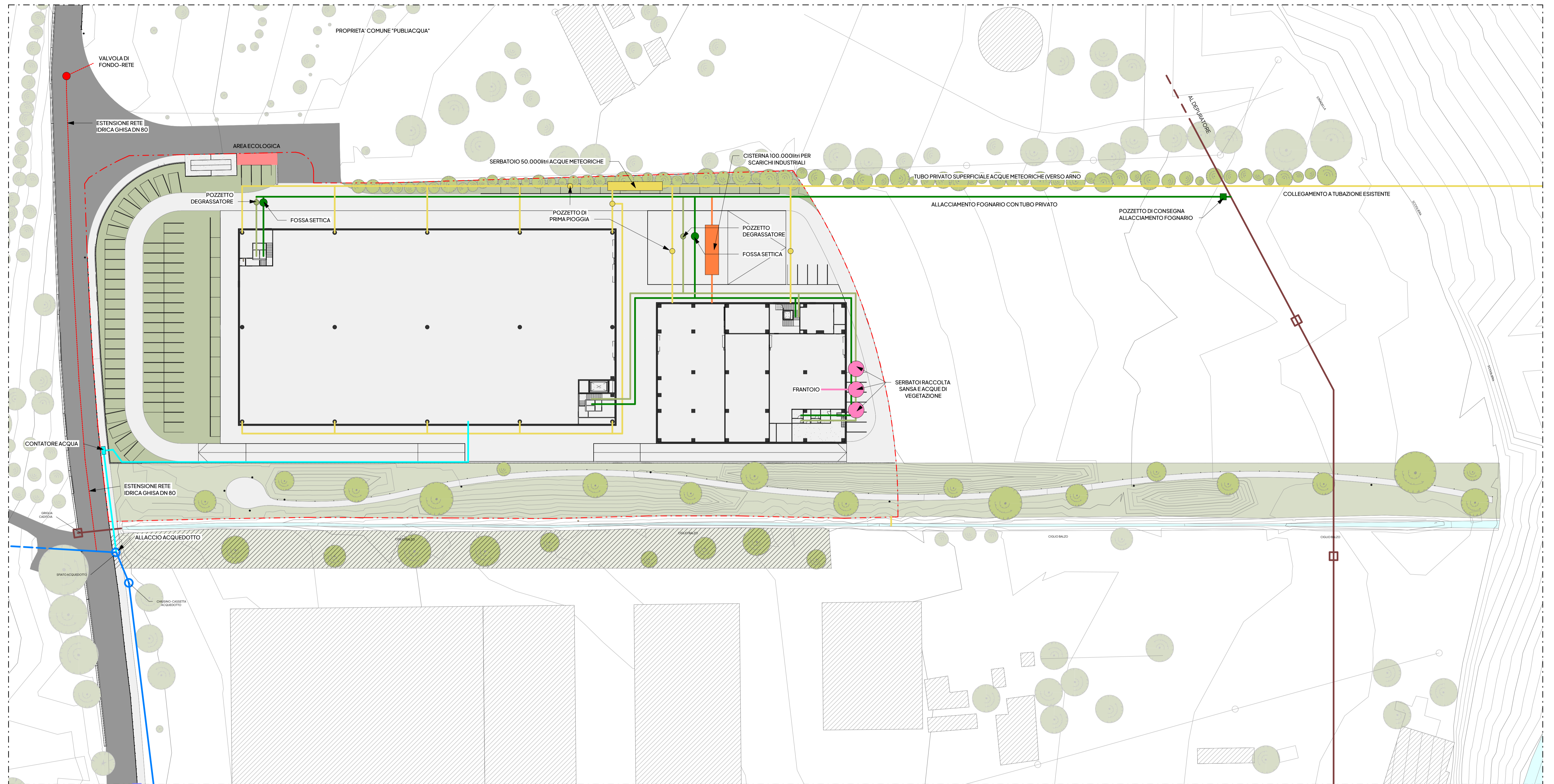
SOTTOSERVIZI SCARICHI E ADDUZIONI _ 1:500
