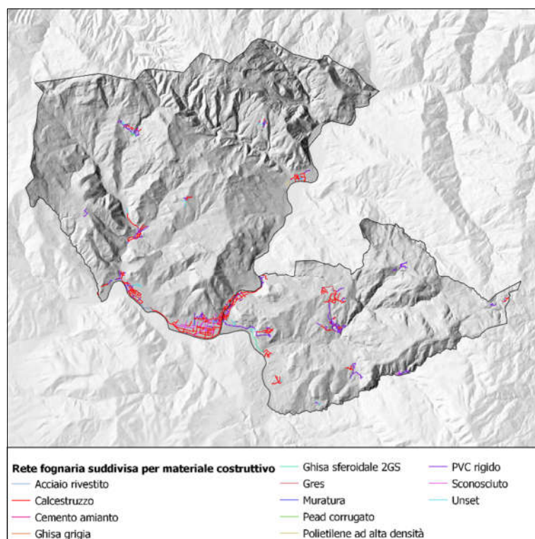
Figura 116 – Estensione rete fognaria suddivisa per materiale costruttivo (Fonte: Publiacqua s.p.a., modificati)
