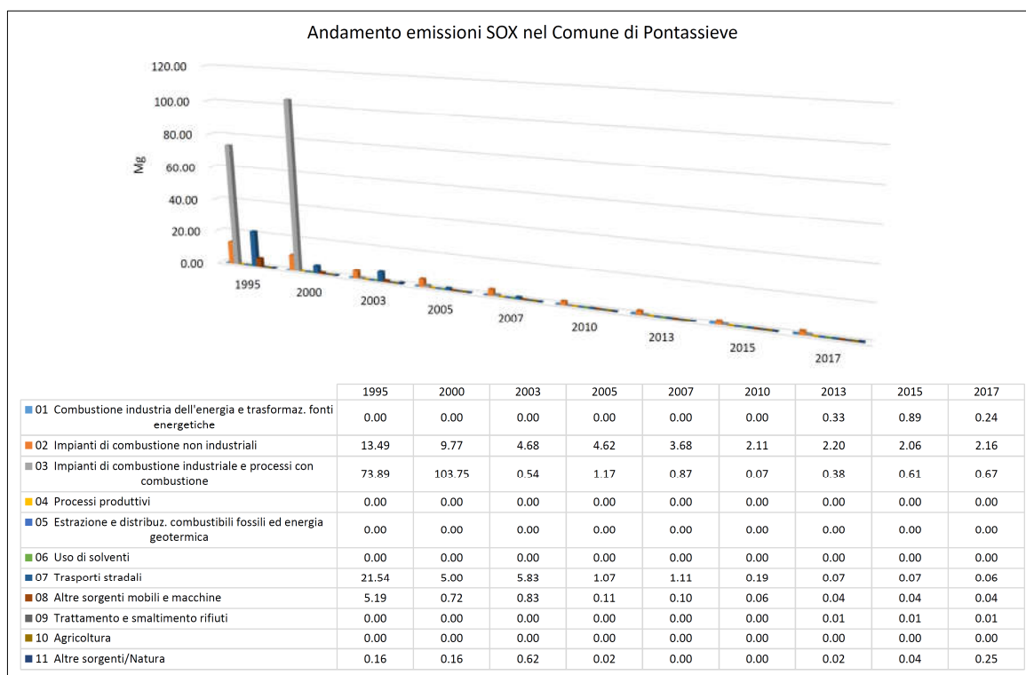
Figura 132 – Emissioni SOX, Comune di Pontassieve. Fonte: IRSE
