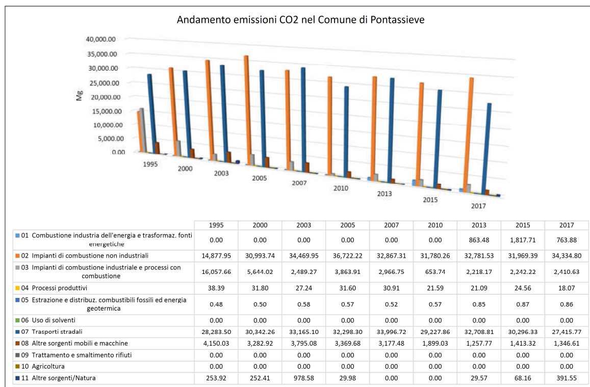
Figura 125 – Emissioni CO2, Comune di Pontassieve. Fonte: IRSE
