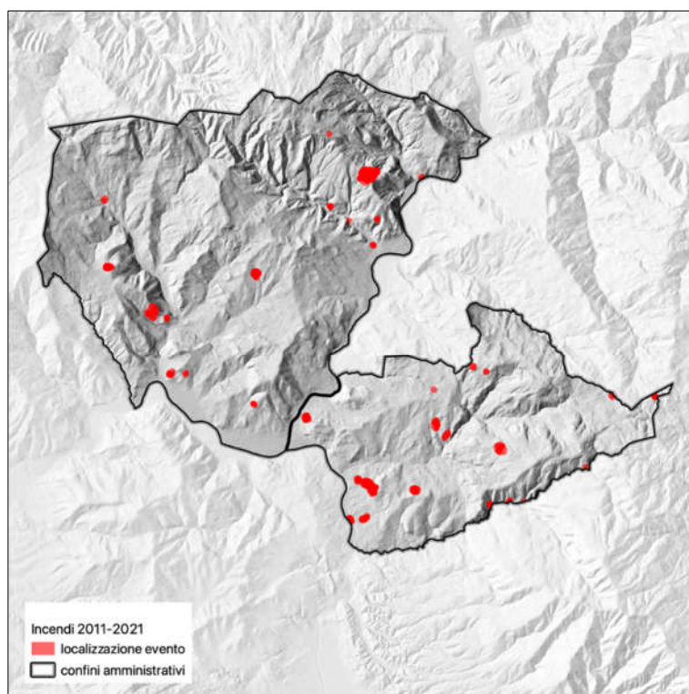
Figura 154 - Localizzazione degli incendi nel territorio del PSI nel decennio 2011-2021
